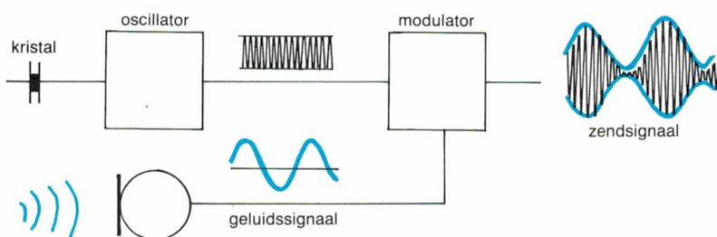
Fig. 1 Principe van AM modulatie
