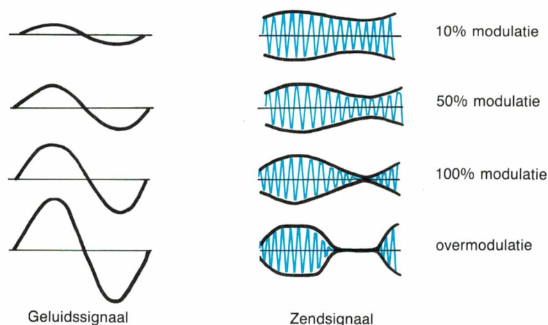
Fig. 2 Modulatiediepte
